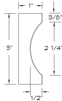
45° CORNER FILLER
