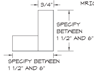
RISER MOULDING
