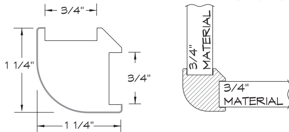
90° CORNER FILLER
