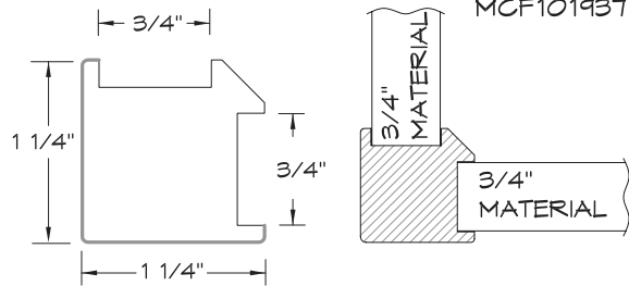
90° CORNER FILLER
