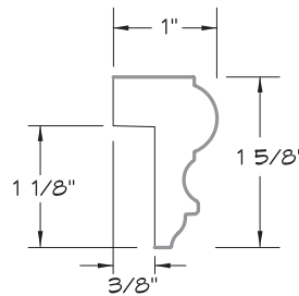
RISER MOULDING
